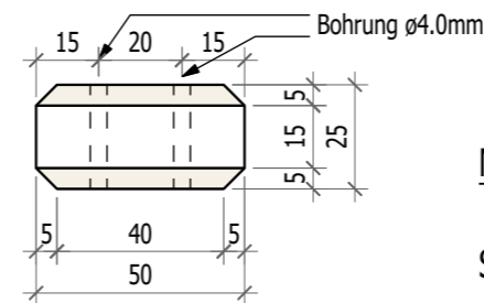
Seitenansicht
