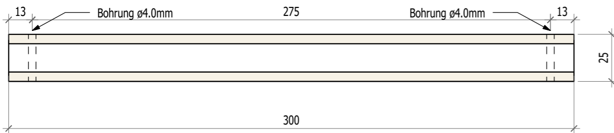
Frontansicht
